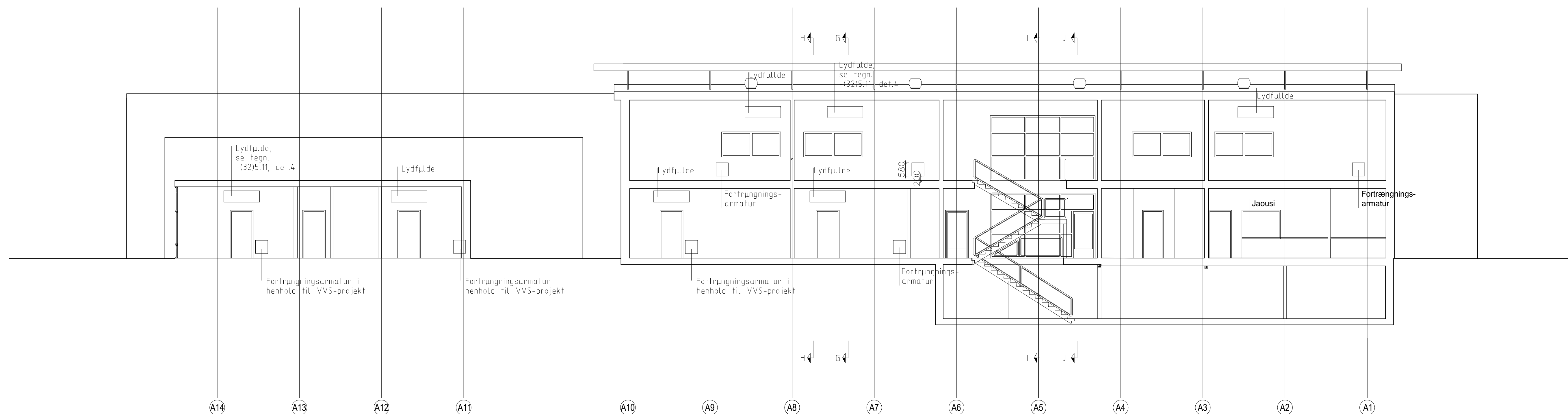
LÆNGDESNIET E-E, OPSTALT SKRÅ VÆG INDEFRA
